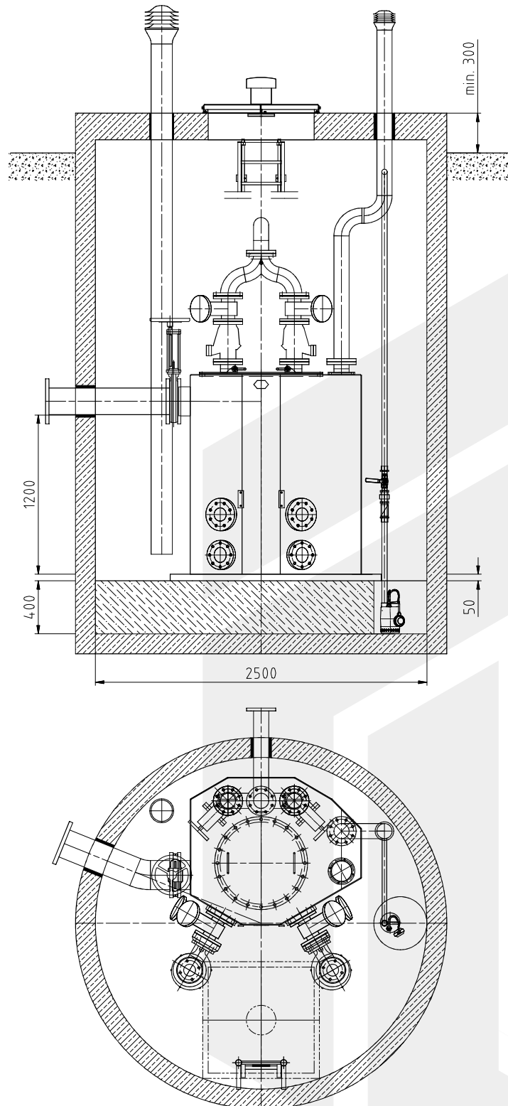
Rysunek przykładowej zabudowy tłoczni ścieków PK35 w komorze
