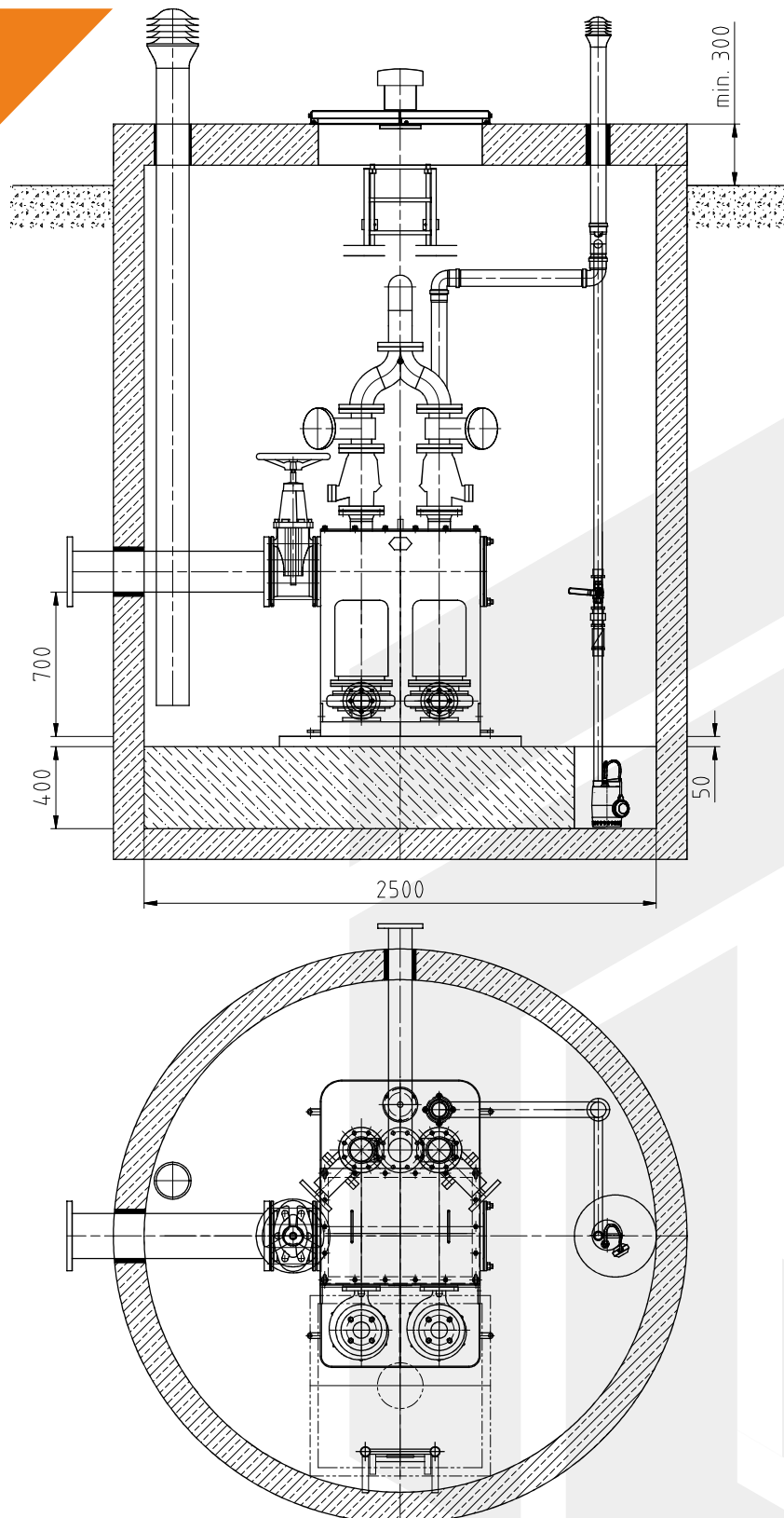
Rysunek przykładowej zabudowy tłoczni ścieków PK15 w komorze
